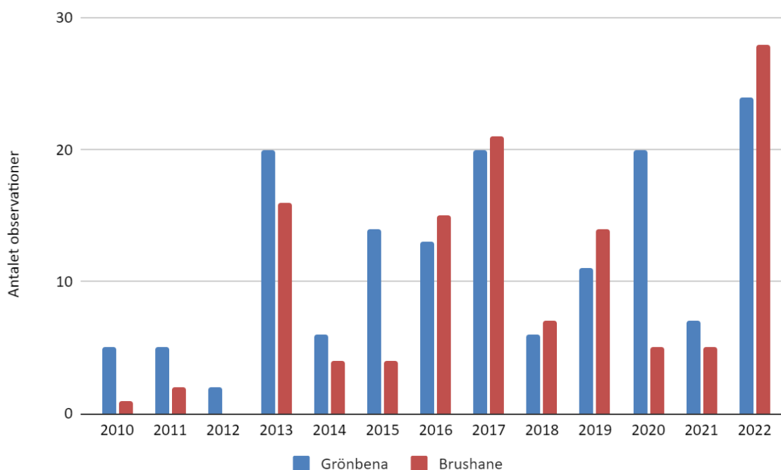
Figur 1. Observationer av grönbena och brushane vid Avasältan och Snötippen 2010-2022 i maj-juni. Brushane har ökat kraftigt 2022 jämfört tidigare år. Båda arterna är arter utpekade för Natura 2000-området Testeboås delta. Diagrammet baseras på data från Artportalen perioden maj-juni under åren 2010-2022.
